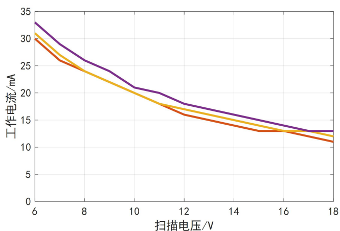
图7-3. 125℃工作电流曲线
