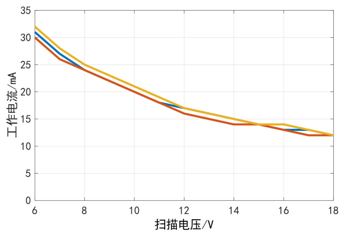
图7-2. 25℃工作电流曲线
