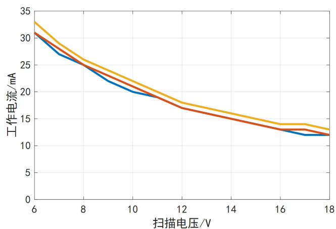
图7-1. -40℃工作电流曲线
