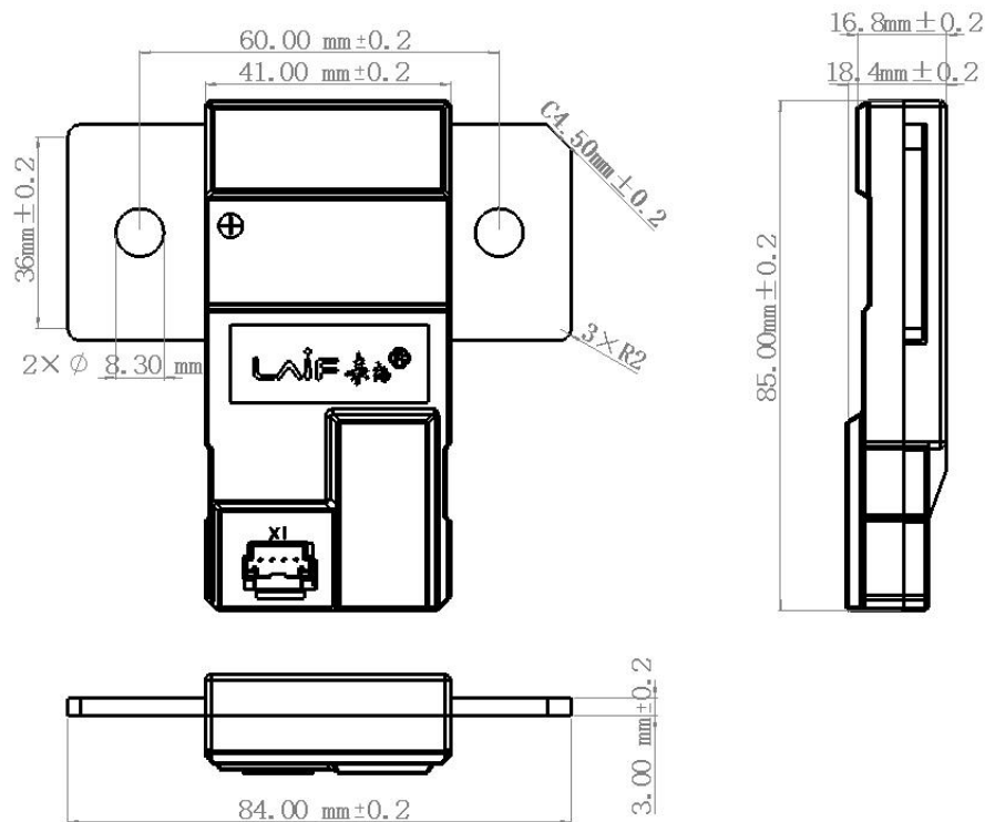
图10-1. 电流传感器外形尺寸示意图
