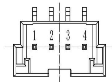
图10-3. 连接器
