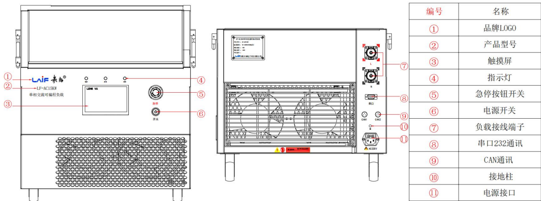
7-1 设备外观图
