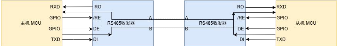
图8-1. RS-485数据链路示意图
